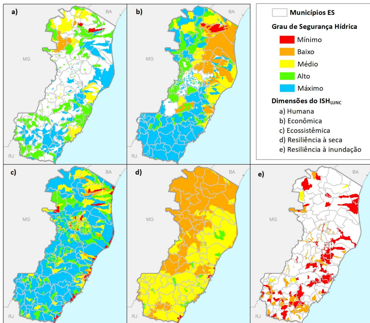
Figura 16. Índice de segurança hídrica no estado do Espírito Santo para o ano 2020 nas dimensões (a) humana, (b) econômica, (c) ecossistêmica, (d) resiliência à seca e (e) resiliência à inundaç o.
